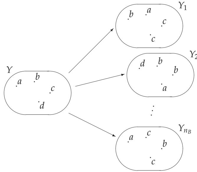
FIGURE 4.2: Illustration de la création des ensembles de bootstrap.
