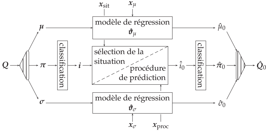
FIGURE 5.8: Schéma de notre méthode de prédiction.
