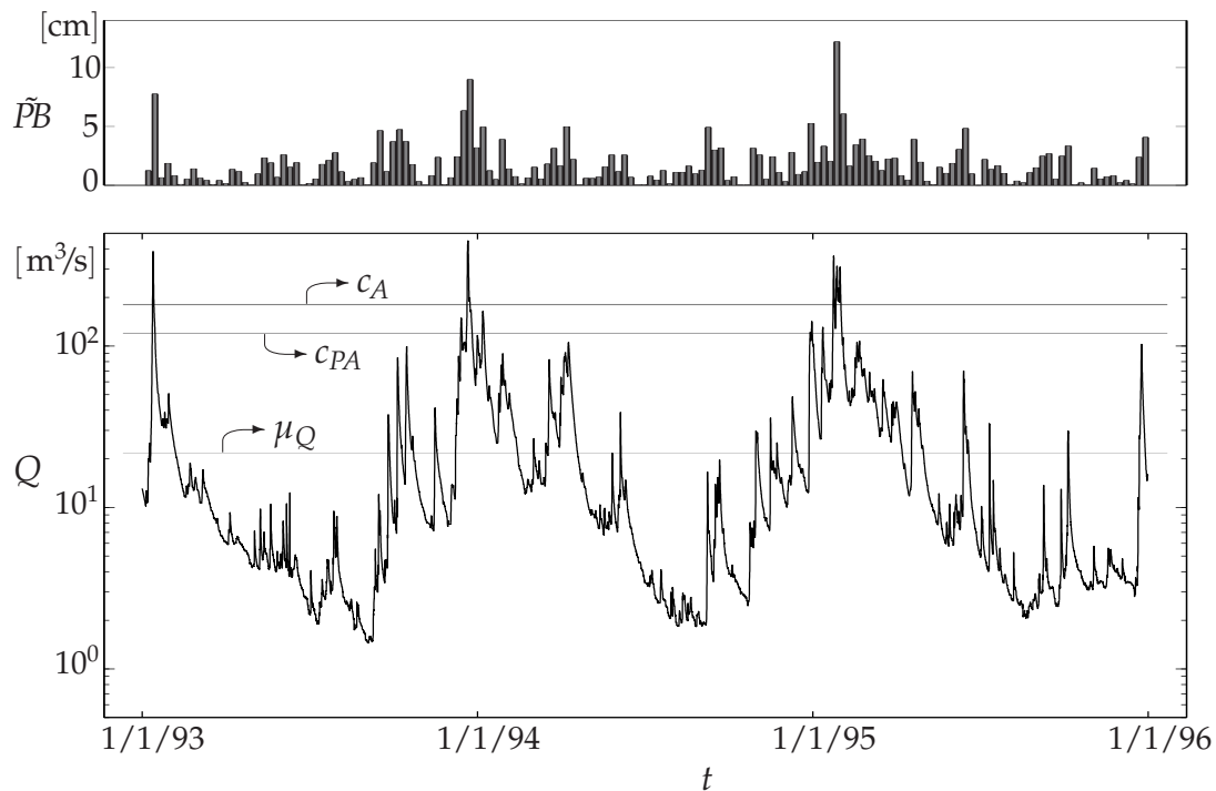
FIGURE 2.3: Mesures de débit à Gendron et la pluie brute (par semaine).
