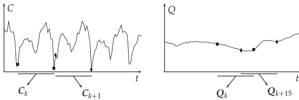
FIGURE 5.3: Construction des courbes de consommation d'électricité et des courbes de débit.
