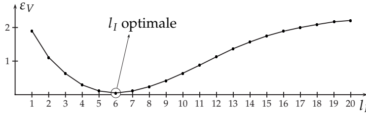
FIGURE 5.4: Illustration de la sélection du nombre d'éléments dans I .
