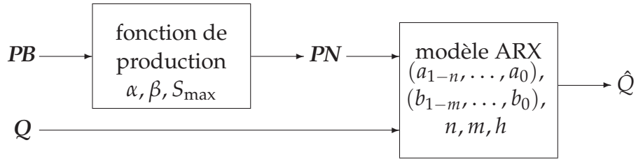
FIGURE 5.1: Schéma du modèle Hydromax.
