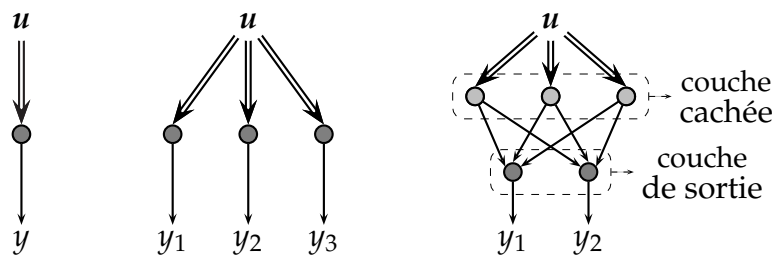
FIGURE 3.5: Trois architectures : le neurone simple, le réseau mono-couche et le réseau multi-couches.
