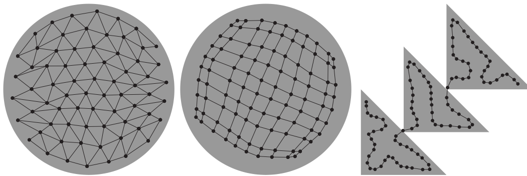
FIGURE 3.15: Encore quelques cartes auto-organisatrices.
