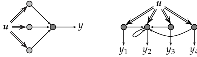
FIGURE 3.6: Schémas des réseaux RBF et SOM.
