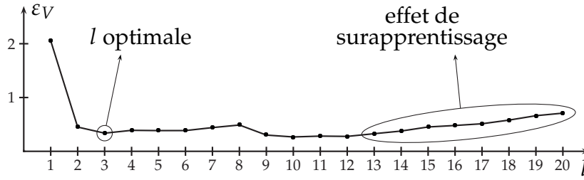
FIGURE 4.3: Illustration de la sélection de la longueur du régresseur.
