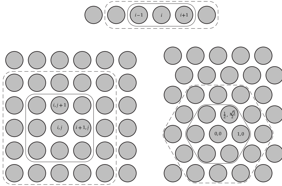
FIGURE 3.10: Trois structures de centroïdes et exemples de voisinages.
