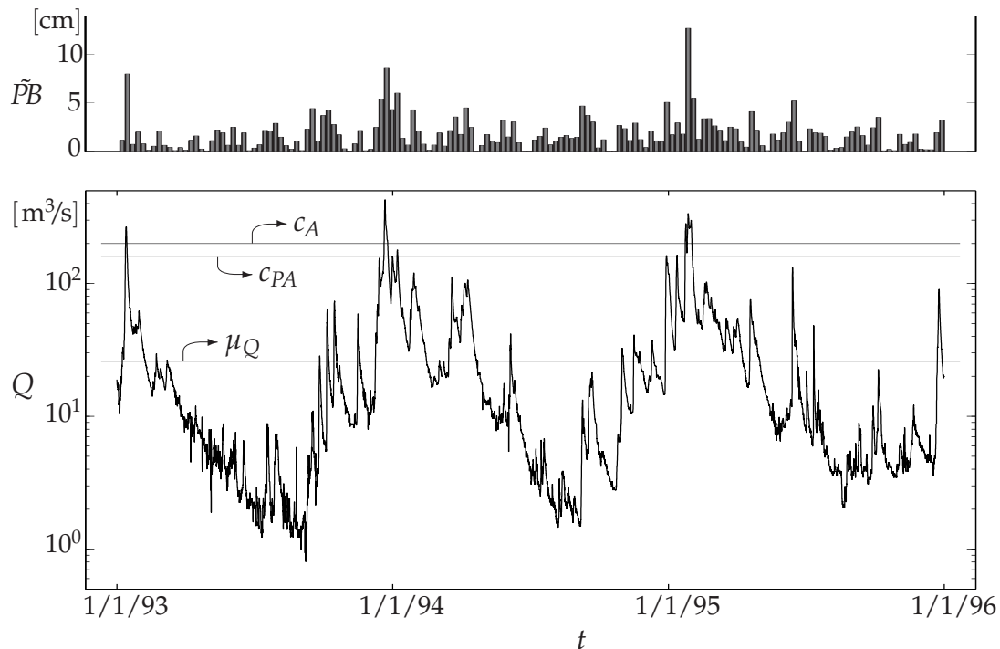
FIGURE 2.4: Mesures de débit à Tabreux et la pluie brute (par semaine).
