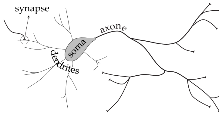
FIGURE 3.1: Le neurone biologique.
