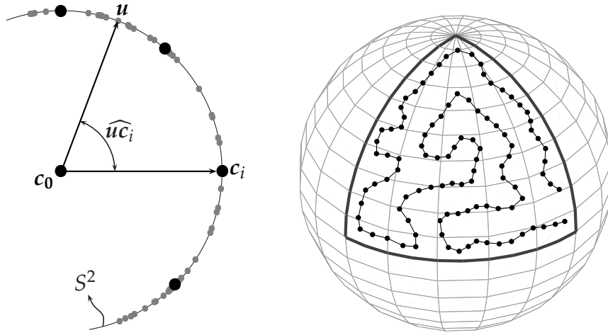
FIGURE 3.16: Illustration des cartes auto-organisatrices à produit scalaire.
